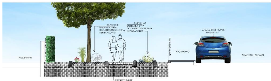
Λεπτομερής τομή
