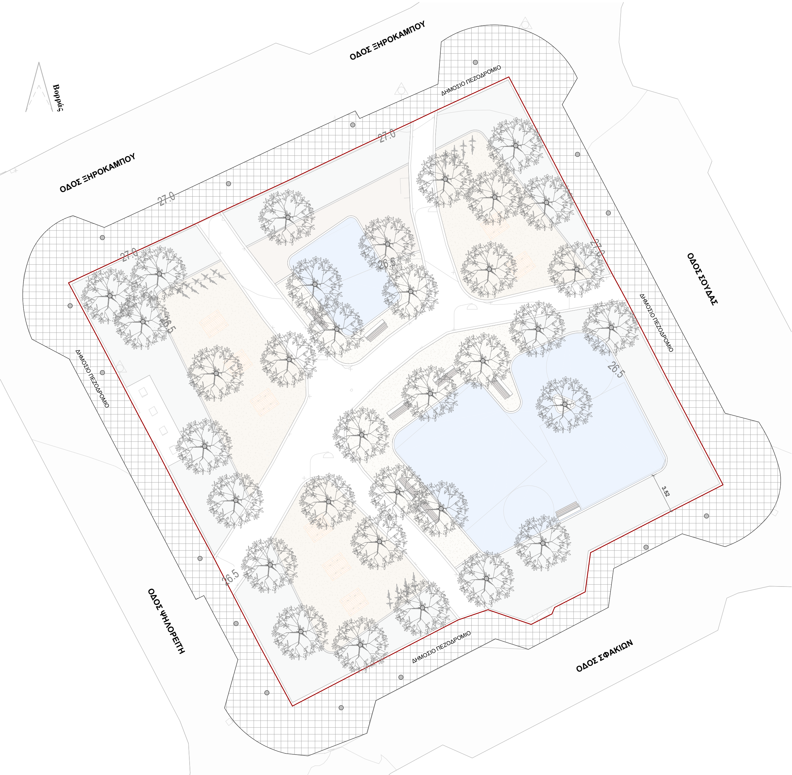
ΠΑΡΚΟ Ε - ΟΔΟΣ ΞΗΡΟΚΑΜΠΟΥ_ ΤΕΜ.346 ΥΦΙΣΤΑΜΕΝΗ ΦΥΤΕΥΣΗ ΚΛ. 1:200
